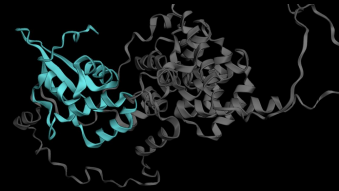
2. DDBH1
